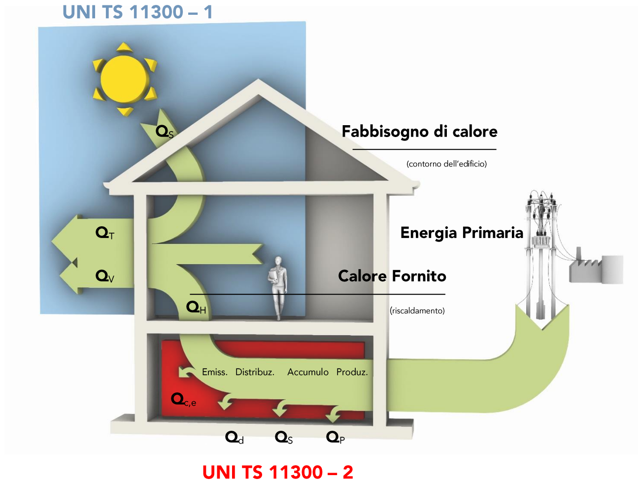
Figura 4 Concettualizzazione del bilancio energetico di un edificio tipo - Fonte: Candidato
