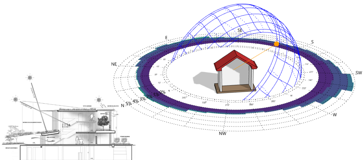
Figura 8 Esposizione solare e diagramma del sole e dei venti in un'analisi ambientale - Fonte: Candidato
