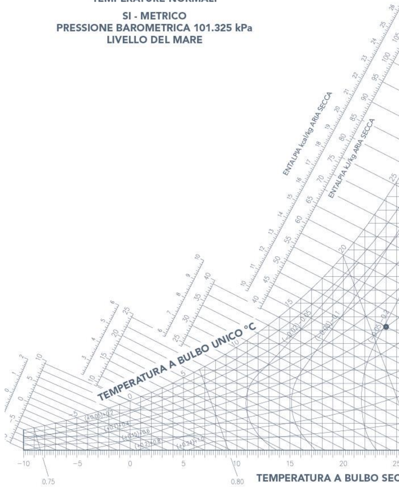
Figura 10 Diagramma Psicrometrico - Fonte: Dispensa Corso di Fisica Tecnica Prof. Dall'O - Politecnico di Milano 2023
