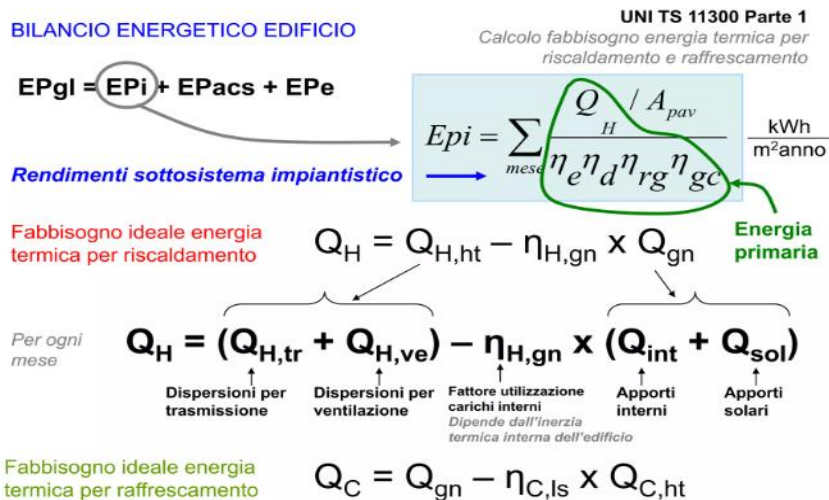
Figura 9 Espressione raffigurante il calcolo del fabbisogno energetico di un edificio - Fonte: Dispense corso di aggiornamento per Certificatori Energetici Collegio Geometri e Geometri laureati di Monza e della Brianza - luglio 2024
